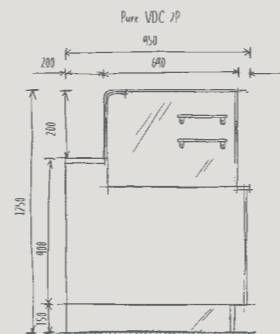
Vitrine totalmente refrigerada com 2 prateleiras. Fully refrigerated showcase with 2 shelves. Vitrine entièrement réfrigérée avec 2 étagères. Vitrina completamente refrigerada con 2 estantes.
