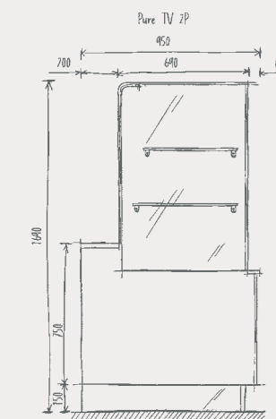
Torre de exposição neutra. Neutral tower exposition. Tour d'exposition neutre. Torre de exhibición neutra.
