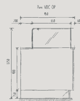
Vitrine totalmente refrigerada sem prateleiras. Fully refrigerated showcase without shelves. Vitrine entièrement réfrigérée sans étagères. Vitrina completamente refrigerada sin estantes.
